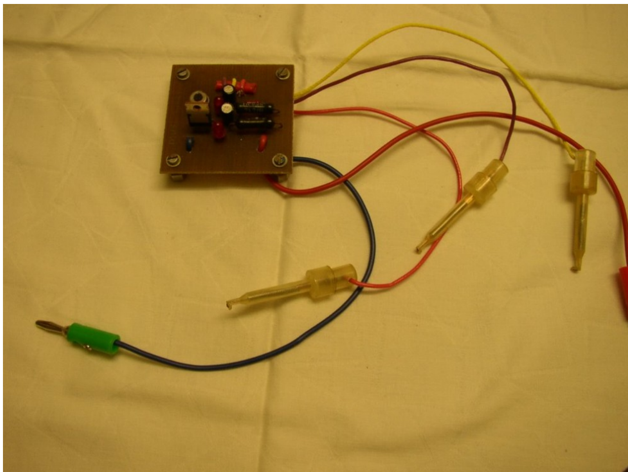
Tester tranzistorů shotky – výkonové.JPG
