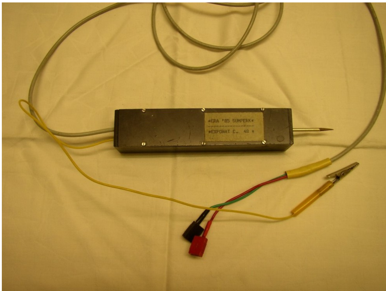
ERA Šumperk – tester IO TTL 85r..JPG
